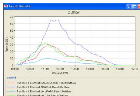
Hidrogramas generados por HEC-HMS de la Cuenca Alta del Rio san Cristóbal—Bogotá DC
