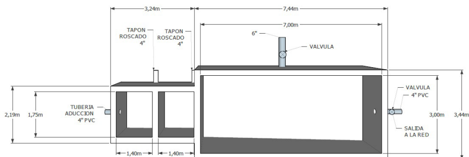
Figura 1. Desarenador actual (vista en planta)
