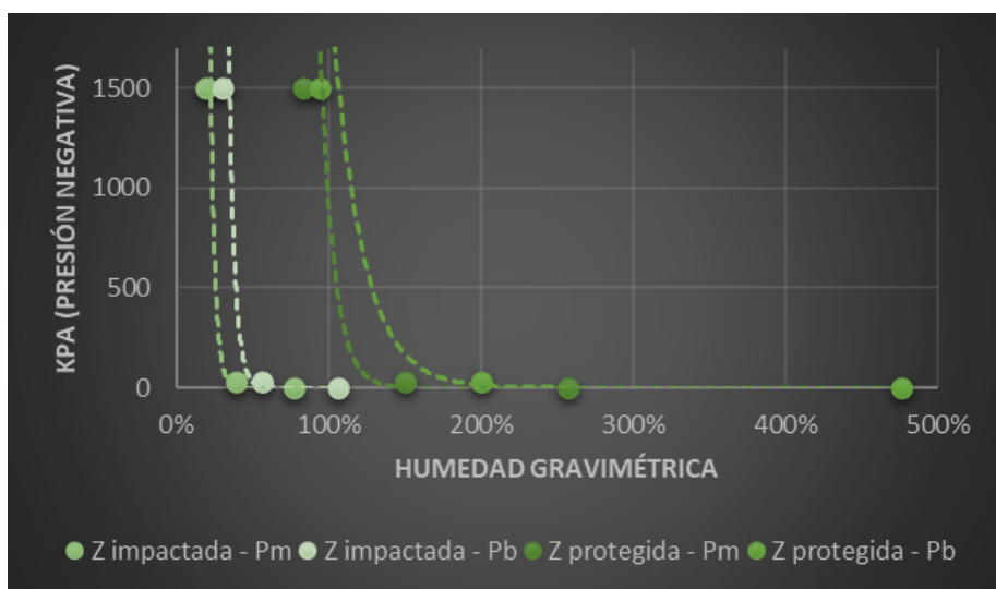
Figura 2. Curvas de retención hídrica para las zonas estudiadas
